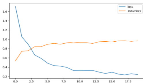
Rys. 2. Krzywa konwergencji z treningu sieci
