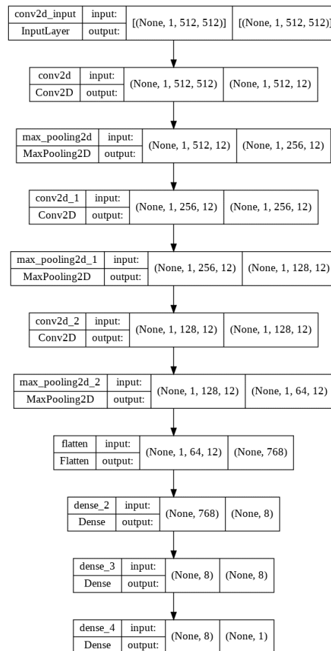
Rys. 3. Architektura wykorzystanej sieci neuronowej
